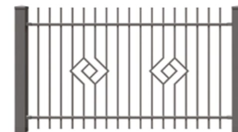
PRZĘŚŁO PROSTE (TYP P) Maksymalna dostępna szerokość: 3000 mm Minimalna standardowa szerokość: 2000 mm
